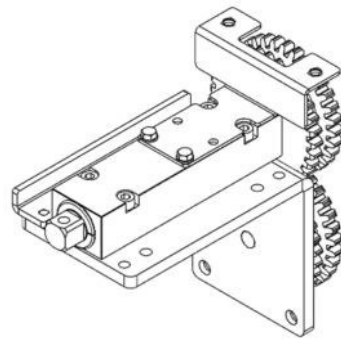
Seitliche Antriebsgruppe links
