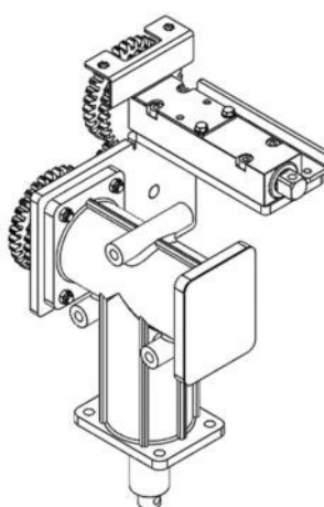
Manuelle seitliche Antriebsgruppe rechts
