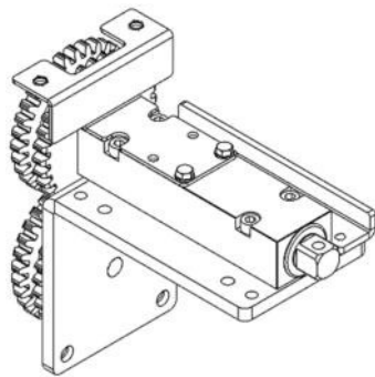
Seitliche Antriebsgruppe rechts
