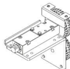
Seitliche Antriebsgruppe links
