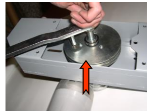
6 Notfallkurbel in der Mitte der Antriebswelle anschrauben. Vorsicht: Runden Stift in den geeigneten Sitz hineinstecken.
