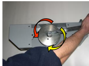
8 Jetzt sind die Antriebswelle und das Untersetzungsgetriebe von der Umlenkrolle entblockt und man kann mit dem manuellen Antrieb der Abdeckung fortfahren.
